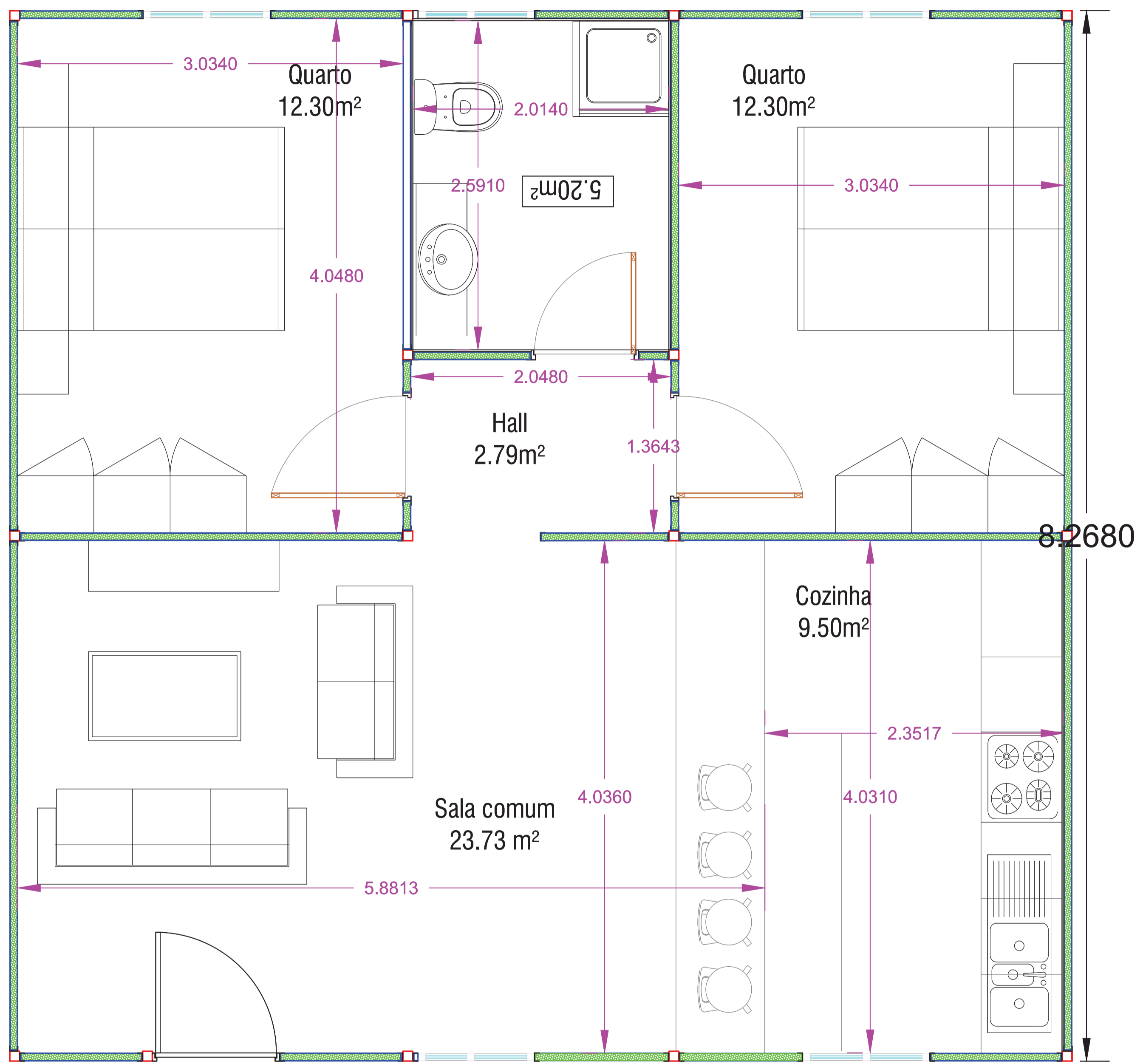
Planta Piso
